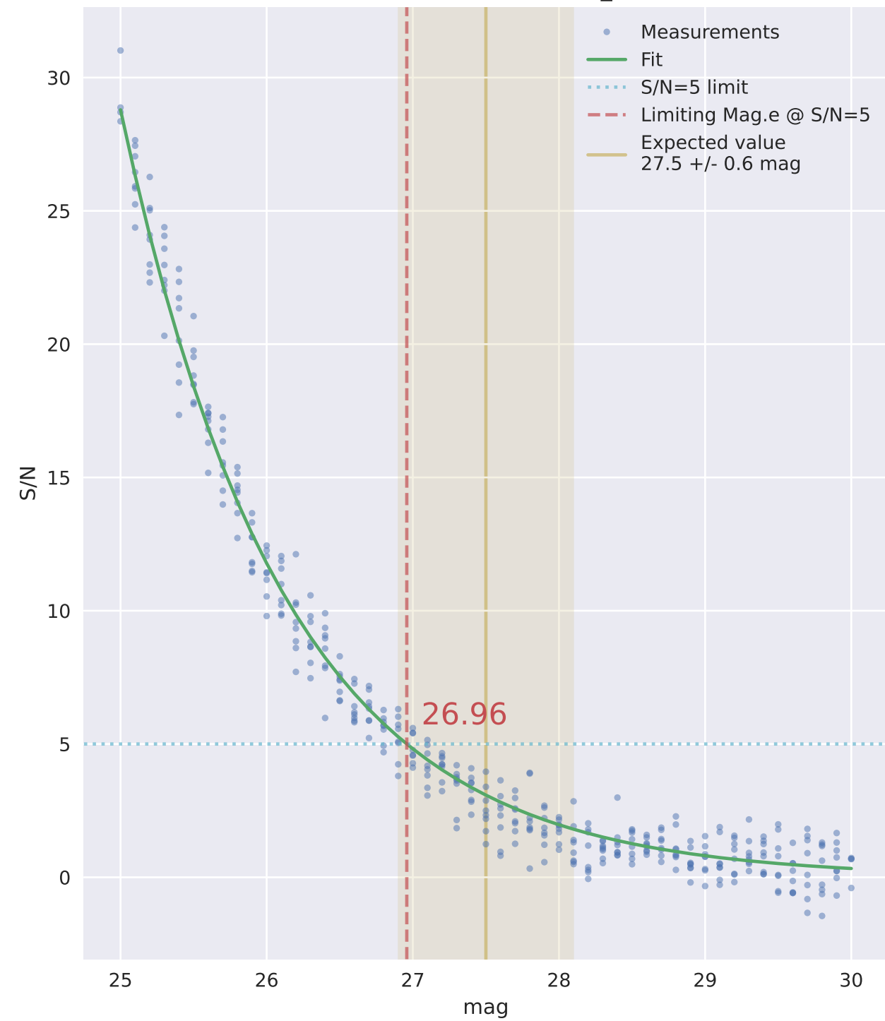
S/N for MICADO MCAO IMG_4mas
